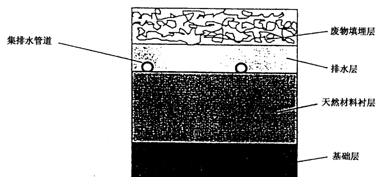
图 3 天然材料衬层示意图
