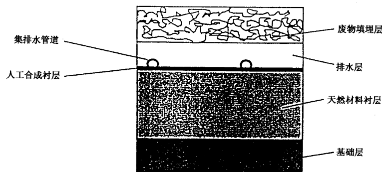
图 2 复合衬层示意图
