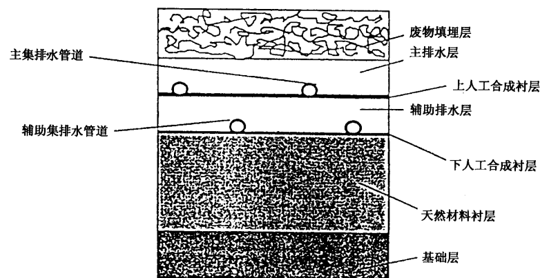
图 1 双人工衬层示意图
